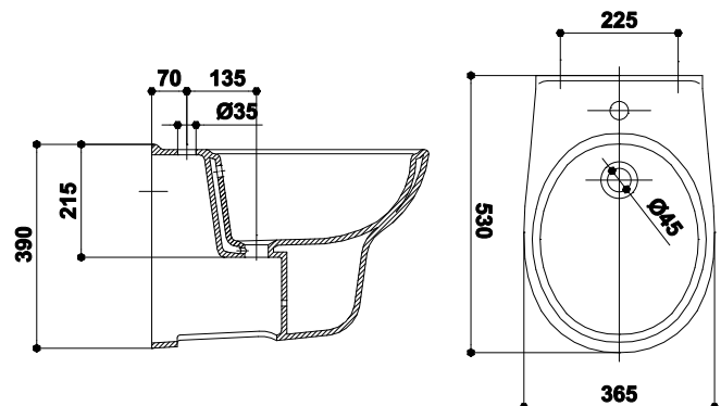
BIDEU SUSPENDAT WALL HANGED BIDET ВЗВЕШЕННЫЙ БИДЕ
