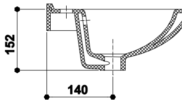
LAVOAR LG WASHBASIN LG РАКОВИНА ЛГ
