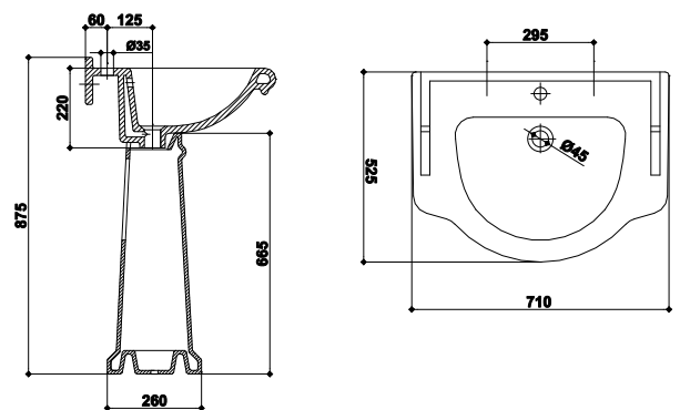
LAVOAR CU PIEDESTAL WASHBASIN WITH PEDESTAL РАКОВИНА С ПЬЕДЕСТАЛОМ
