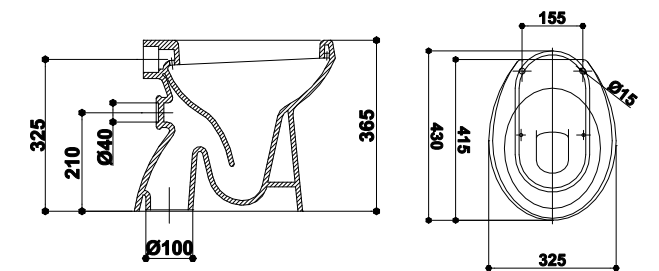
VAS WC REDUS WC BOWL REDUS ТУАЛЕТ РЕДУС
