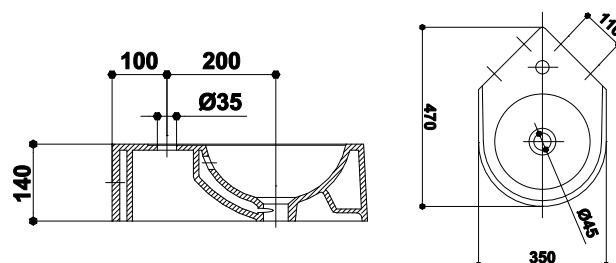
LAVOAR JASMIN WASHBASIN JASMIN РАКОВИНА ЯСМИН
