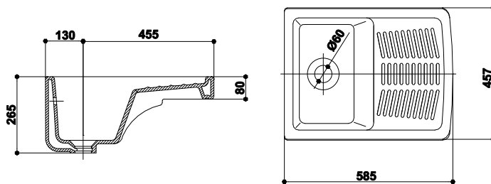
CUVA OLTA WASH TUBE OLTA ВАННА ОЛТА
