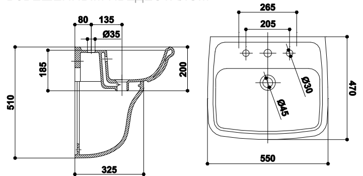
LAVOAR SUSPENDAT WASHBASIN WITH WALL HANGE PEDESTAL РАКОВИНА С ВЗВЕШЕННЫМ ПЬЕДЕСТАЛОМ
