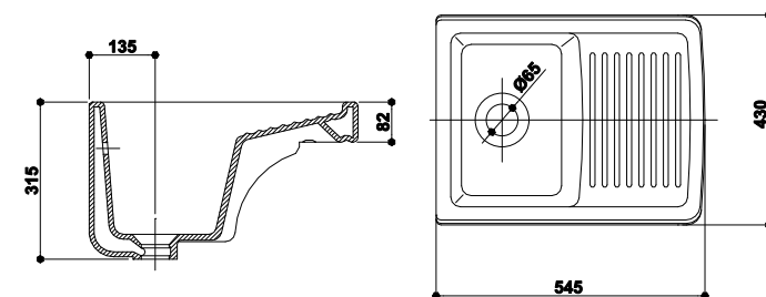
CUVA VOLGA WASH TUBE VOLGA ВАННА ВОЛГА
