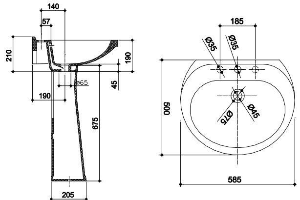
LAVOAR CU PIEDESTAL WASHBASIN WITH PEDESTAL РАКОВИНА С ПЬЕДЕСТАЛОМ
