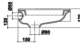
VAS WC TURCESC T6 WC BOWL SQUATTI NG PANT 6 ТУАЛЕТ T6
