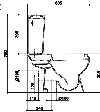
VAS WC MONOBLOC WC BOWL MONOBLOCK ОДНОЧАСТЫЙ ТУАЛЕТ
