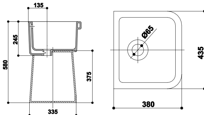
CUVA BIANCA WASH TUBE BIANCA ВАННА БИАНКА
