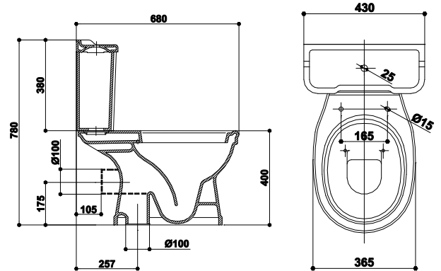
VAS WC MONOBLOC WC BOWL MONOBLOCK ОДНОЧАСТЫЙ ТУАЛЕТ
