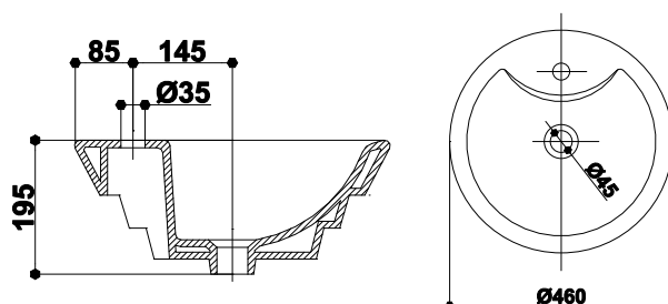
LAVOAR CASCADE WASHBASIN CASCADE РАКОВИНА КАСКАД
