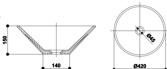
LAVOAR ATHENA WASHBASIN ATHENA РАКОВИНА АТЕНА
