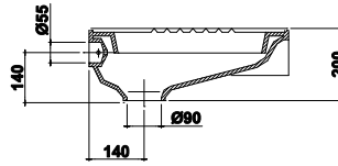
VAS WC TURCESC T5 WC BOWL SQUATTI NG PANT 5 ТУАЛЕТ T5
