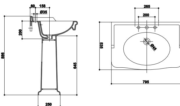
LAVOAR CU PIEDESTAL WASHBASIN WITH PEDESTAL РАКОВИНА С ПЬЕДЕСТАЛОМ
