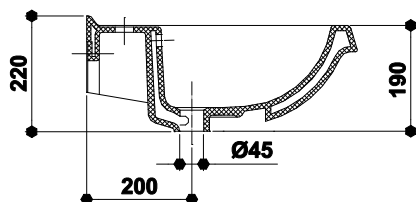
LAVOAR ADRIA WASHBASIN ADRIA РАКОВИНА ТОП АДРИА
