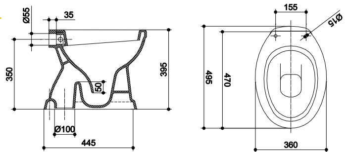
VAS WC NORMAL WC BOWL НОРМАЛЬНЫЙ ТУАЛЕТ
