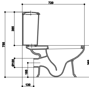
VAS WC MONOBLOC WC BOWL MONOBLOCK ОДНОЧАСТЫЙ ТУАЛЕТ
