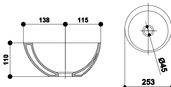
LAVOAR FLORANCE WASHBASIN FLORANCE РАКОВИНА ФЛОРЕНС
