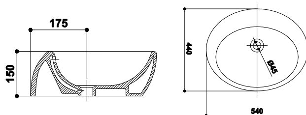
LAVOAR GALICE WASHBASIN GALICE РАКОВИНА ГАЛИС
