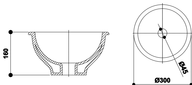
LAVOAR HAWAI WASHBASIN HAWAI РАКОВИНА ГАВАЙИ
