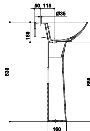
LAVOAR TOPAZIO WASHBASIN TOPAZIO РАКОВИНА ТОПАЦИО
