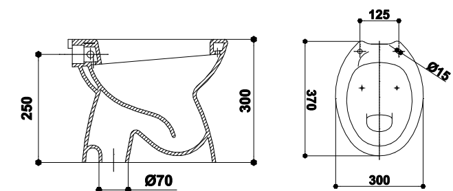
VAS WC CIV CK WC BOWL CIV CK ТУАЛЕТ ЧИВ СК
