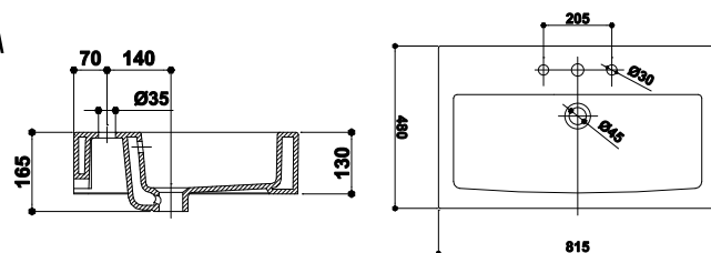
LAVOAR AMPHORA WASHBASIN AMPHORA РАКОВИНА АМФОРА
