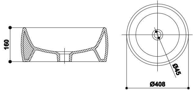
LAVOAR TOP CASTRES WASHBASIN CASTRES РАКОВИНА КАСТРЕС
