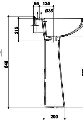
LAVOAR CU PIEDESTAL WASHBASIN WITH PEDESTAL РАКОВИНА С ПЬЕДЕСТАЛОМ
