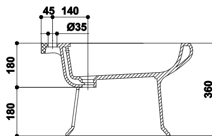
BIDEU BIDET БИДЕ
