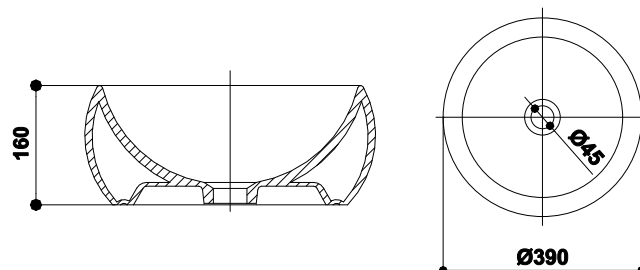
LAVOAR MAYA WASHBASIN MAYA РАКОВИНА МАЙЯ
