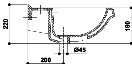
LAVOAR SELENA WASHBASIN SELENA РАКОВИНА ТОП СЕЛЕНА
