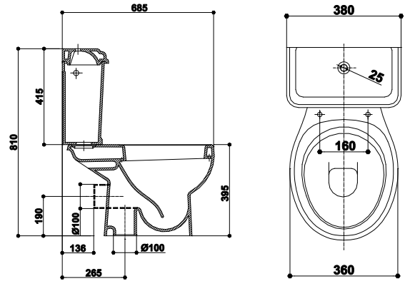
VAS WC MONOBLOC WC BOWL MONOBLOCK ОДНОЧАСТЫЙ ТУАЛЕТ
