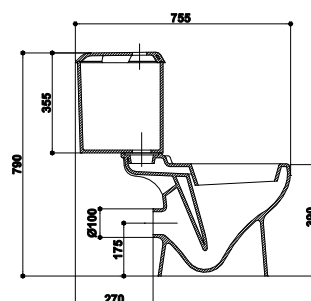
VAS WC MINI CU REZERVOR COLT ANGLE TANK MINI WC BOWL ТУАЛЕТ МИНИ УГОЛНОЙ
