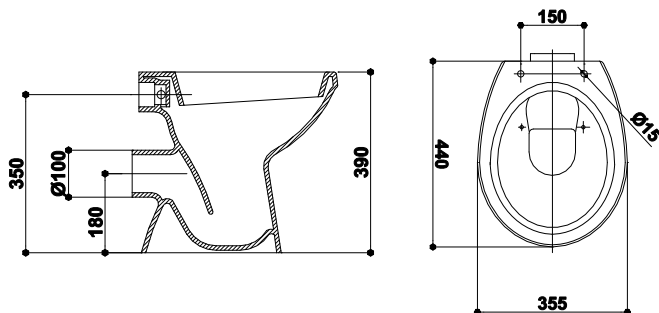
VAS WC CIL/CIV WC BOWL CIL/CIV ТУАЛЕТ ЧИЛ/ЧИВ
