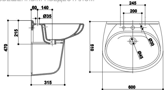
LAVOAR SUSPENDAT WASHBASIN WITH WALL HANGE PEDESTAL РАКОВИНА С ВЗВЕШЕННЫМ ПЬЕДЕСТАЛОМ
