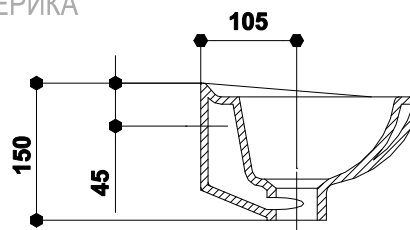
LAVOAR ERIKA WASHBASIN ERIKA РАКОВИНА ЕРИКА
