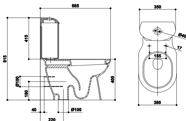
VAS WC MONOBLOC WC BOWL MONOBLOCK ОДНОЧАСТЫЙ ТУАЛЕТ
